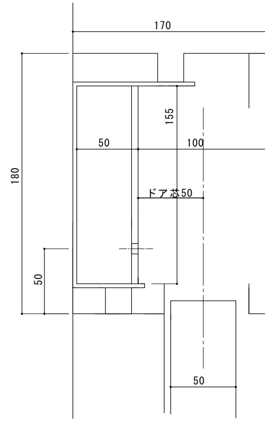
無目断面図
