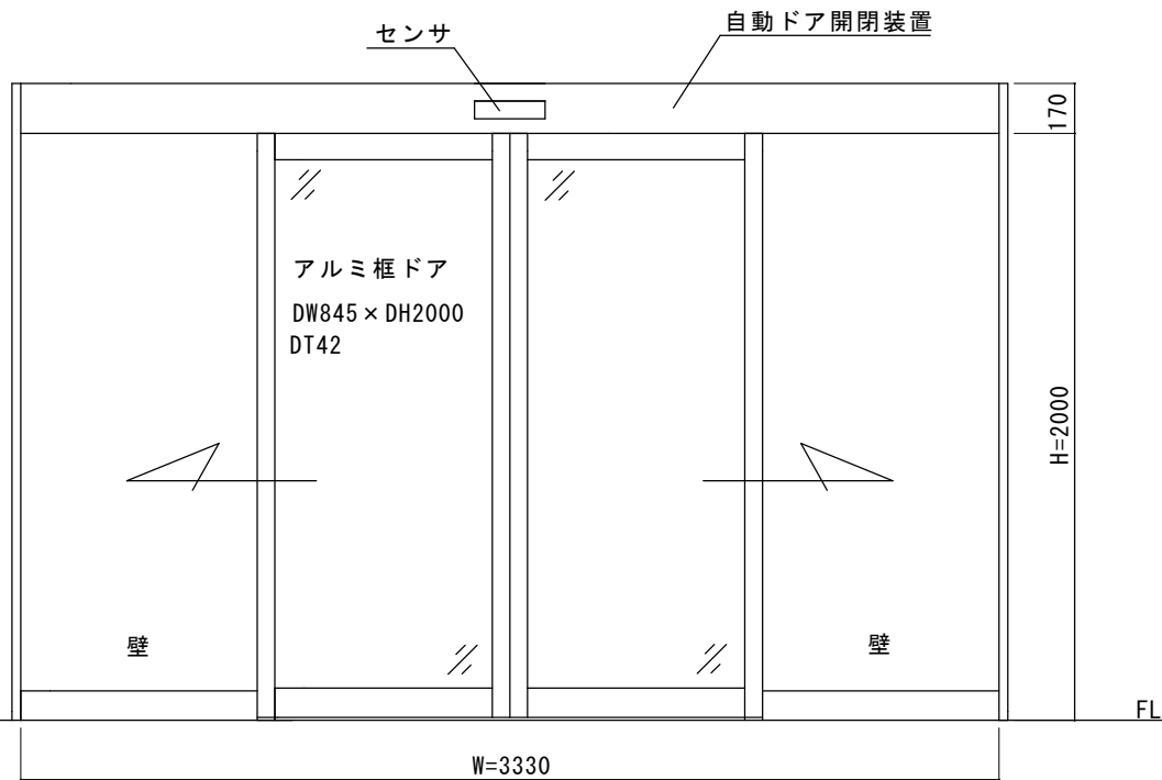
内観図
